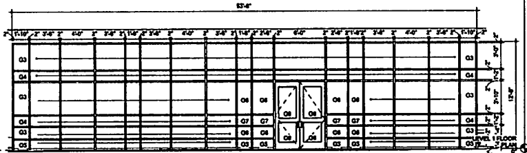
6 FRAME ELEVATION- SF5 SCALE: 1/4" = 1'-0"
