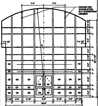
4 FRAME ELEVATION- SF2B SCALE: 1/4" = 1'-0"
